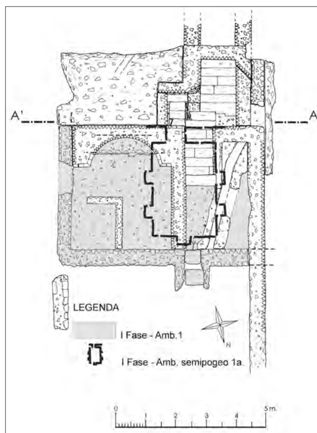
Fig. 4. Palestrina, area 31. I fase con posizionamento del vano seminterrato (ril. D. Raiano, G. Troja, elab. Luigi Carboni).
