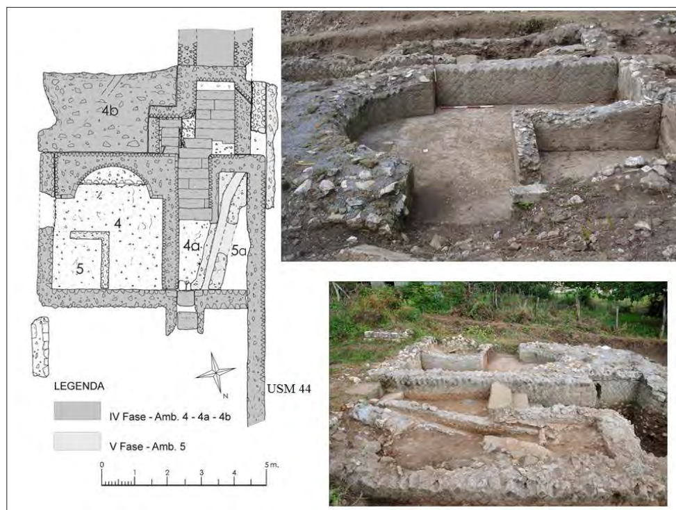
Fig. 9. Area 31. Planimetria della IV e V fase. Ambienti 4 e 5 visti da est e andito 4a, in cui insiste la canaletta 5a, da ovest.
