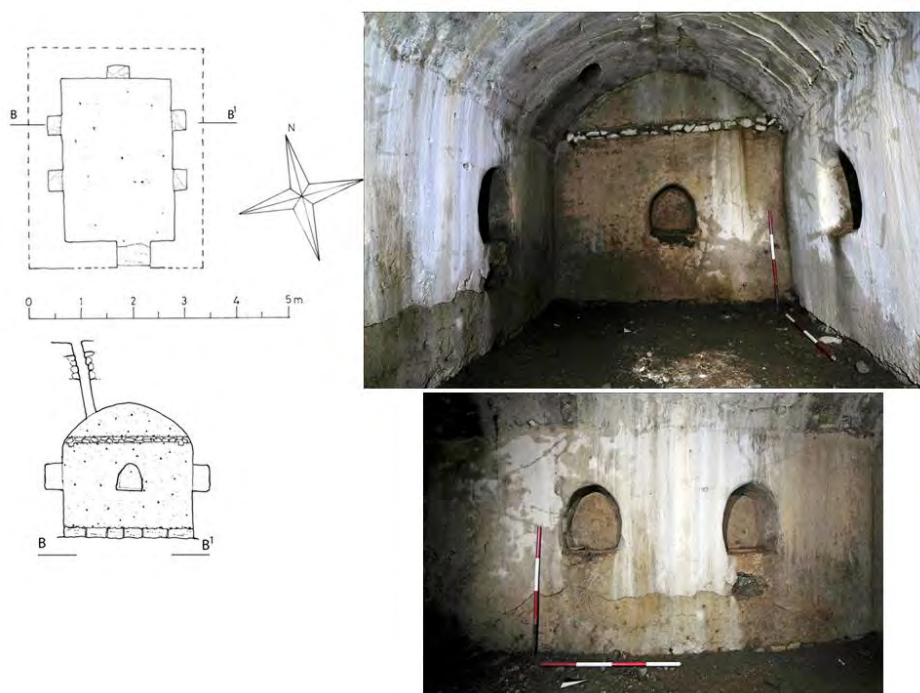
Fig. 6. Planimetria e prospetto dell'ambiente seminterrato 1a (rilievo D. Raiano). Foto generale del vano visto da sud e lato occidentale con nicchie (foto M. Merlo).
