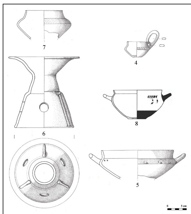
Fig. 2. Corredo fittile della tomba 12 di Colonna, loc. Barberi (disegno C. Predan).
