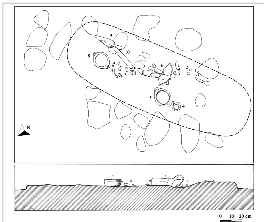
Fig. 1. Pianta e sezione della tomba 12 di Colonna, loc. Barberi (rilievo D. Alfonso).
