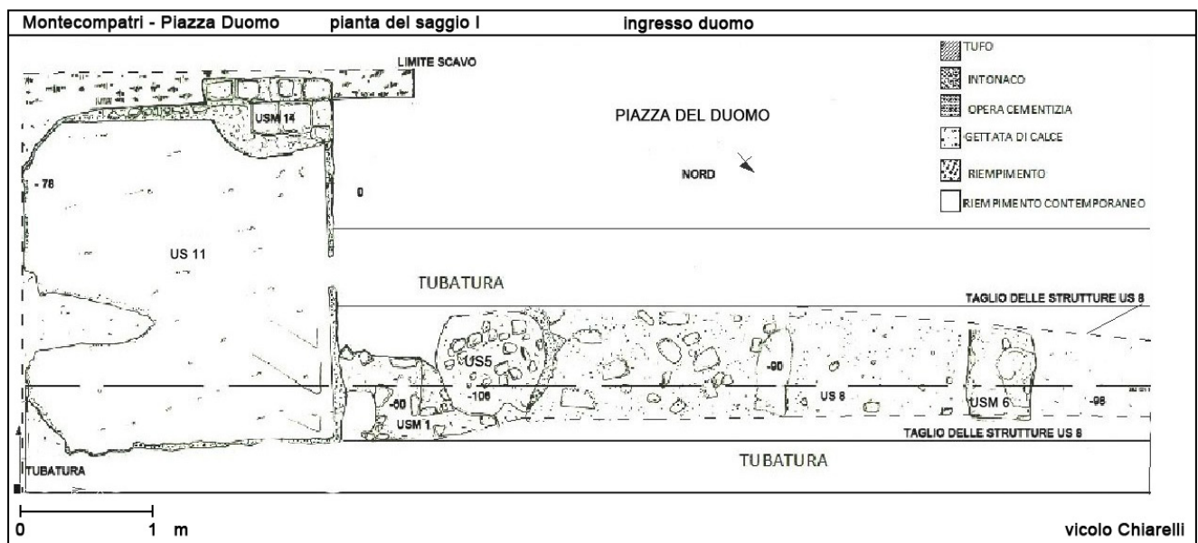
Fig. 1. Pianta del silos e delle strutture accessorie.
